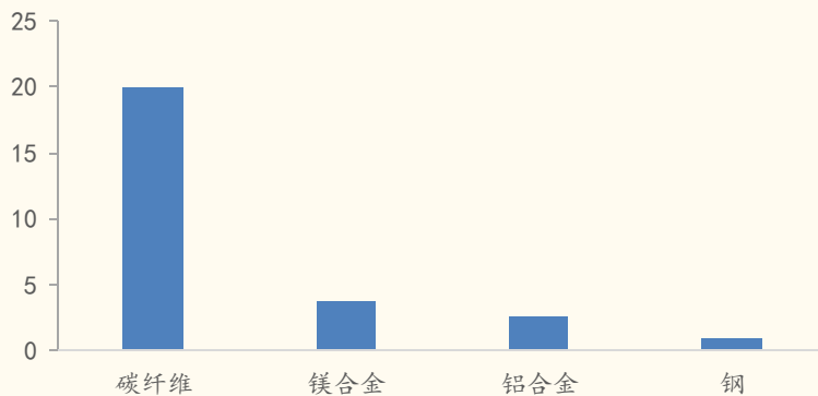
图表 21：碳纤维的轻量化成本最高，镁合金、铝合金次之（美元/kg）
