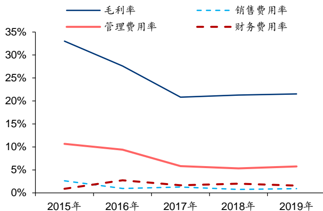
图表2: 2015~2019年毛利率及相关费用率
