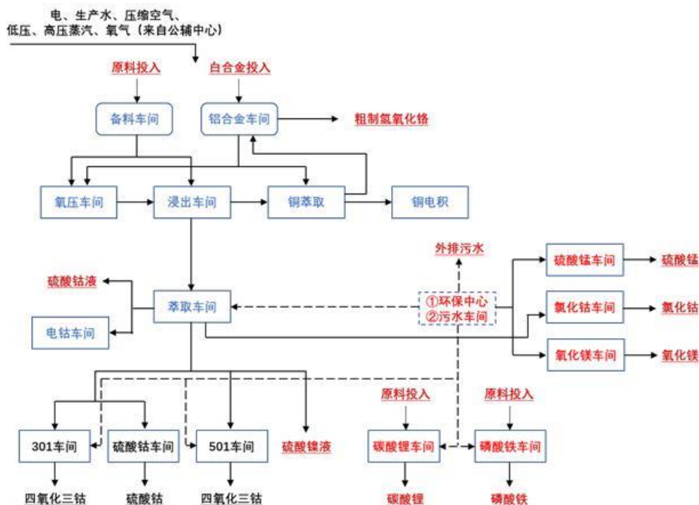
图 15：公司有色板块主要产品工艺流程
