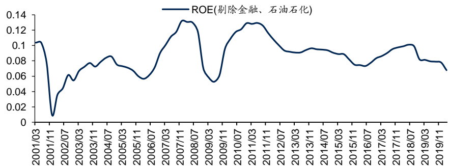
图 48: ROE 走势
