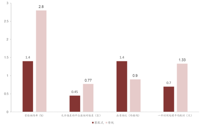
图 29: 工程端装配式和传统装修完工品质实测数据对比
