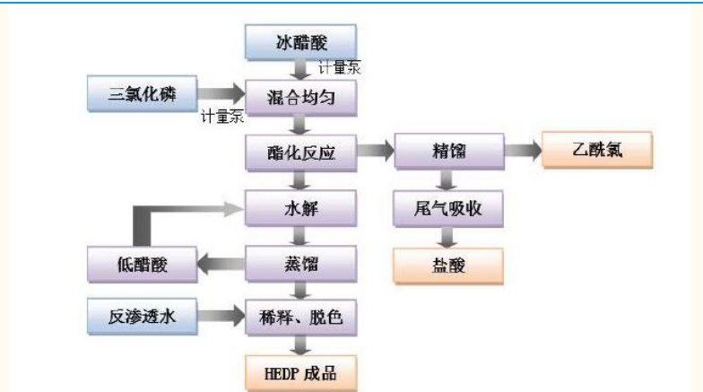
图表 23: HEDP 生产流程图
