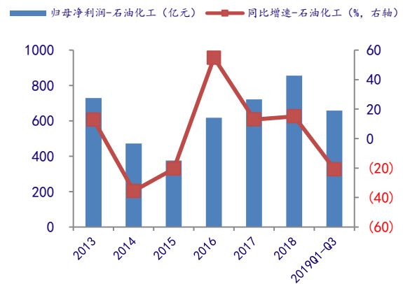
图 19: 石油化工板块归母净利润及增长率
