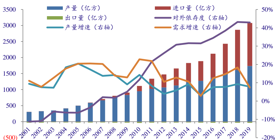
图 8：我国天然气供需及对外依存度
