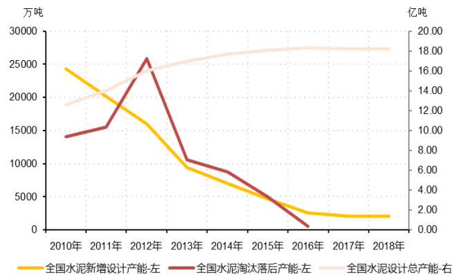
图 9：2010-2019 年水泥产能情况
