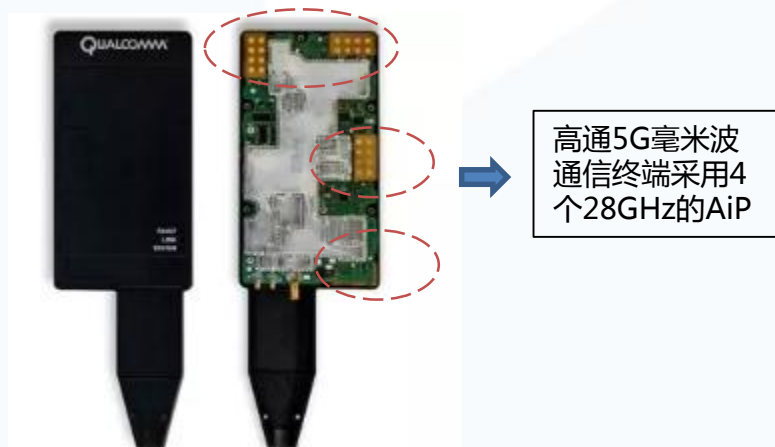
Qualcomm 5G毫米波通信终端参考设计样机
