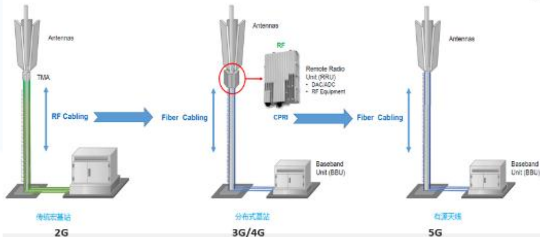
基站的具体形态演化
