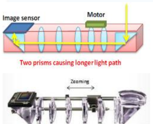
潜望式+马达可实现无级光学变焦
