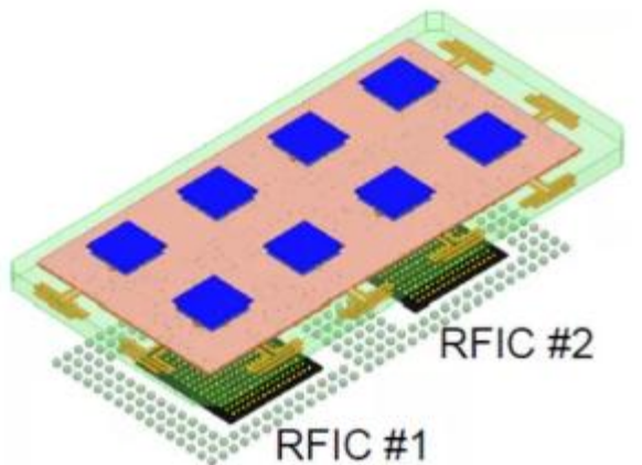
高通5G AiP天线示意图：包含8根天线+2颗射频芯片
