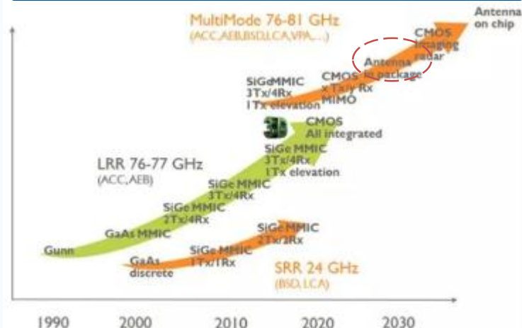
AiP已成为毫米波频段主流天线技术
