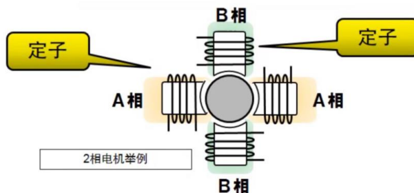
图 7：步进电机根据定子分类
