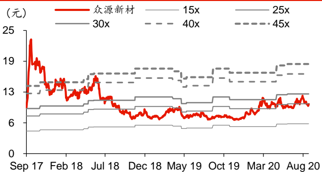
图表4: 众源新材历史 PE-Bands
