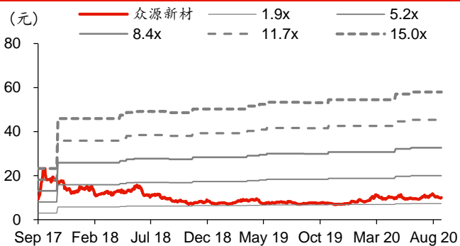
图表5: 众源新材历史 PB-Bands
