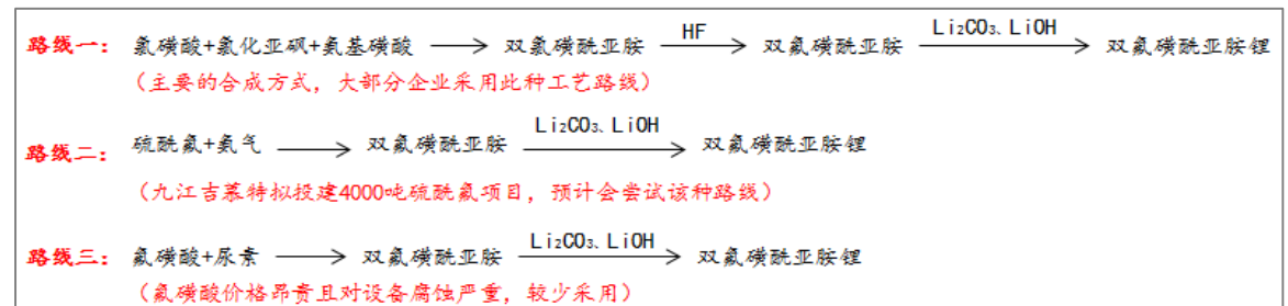
图 33：LiFSI 主要的三种工艺路线
