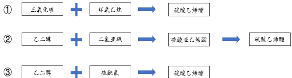
图 30：硫酸乙烯酯生产工艺
