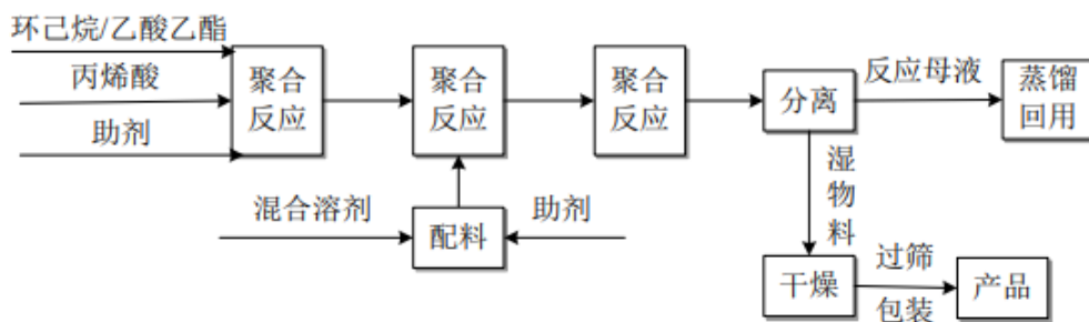
图 42：卡波姆树脂工艺流程图
