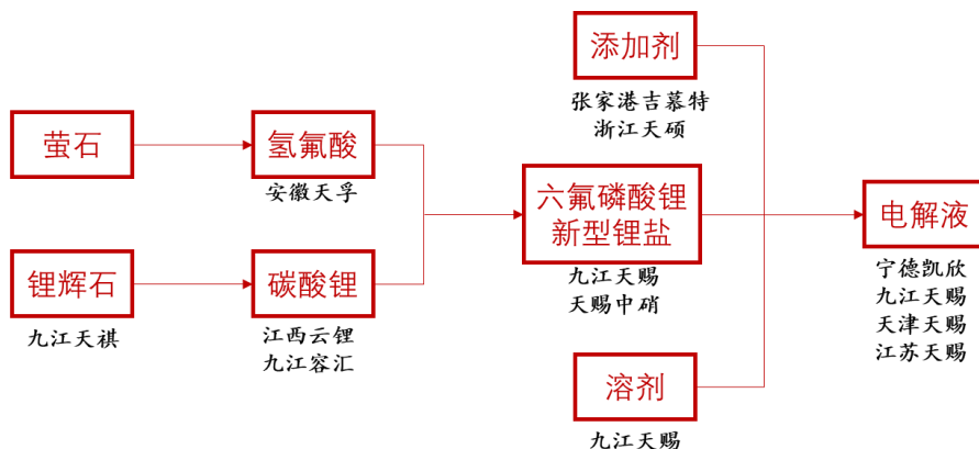
图 13：天赐材料电解液产业链布局
