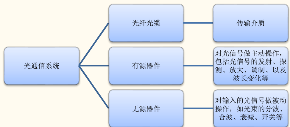
图表 9：光通信系统分类
