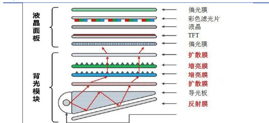
图 1: LED 显示结构
