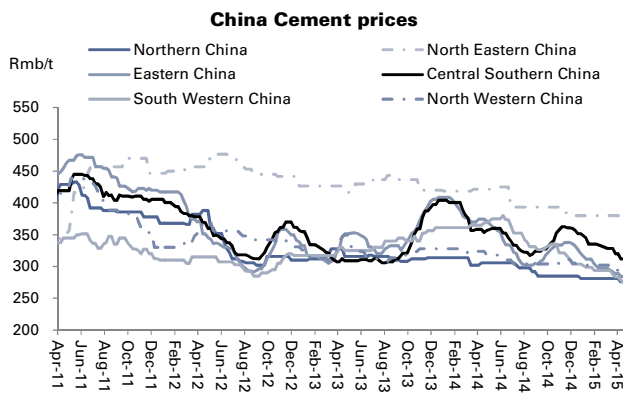
图表2: 中国各地区水泥价格
